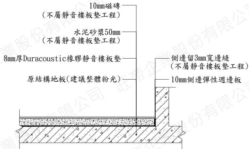
Duracoustic橡膠靜音樓板墊系統剖面圖
