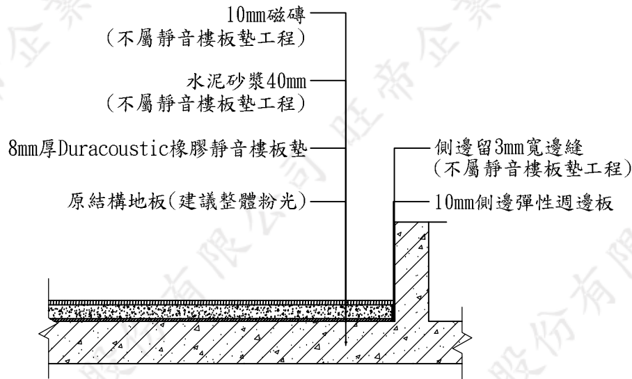
Duracoustic橡膠靜音樓板墊系統剖面圖
